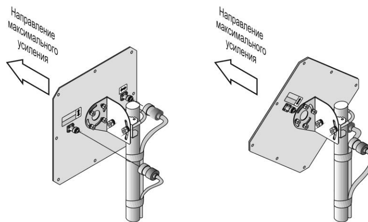
Рисунок 2. Сборка антенны
